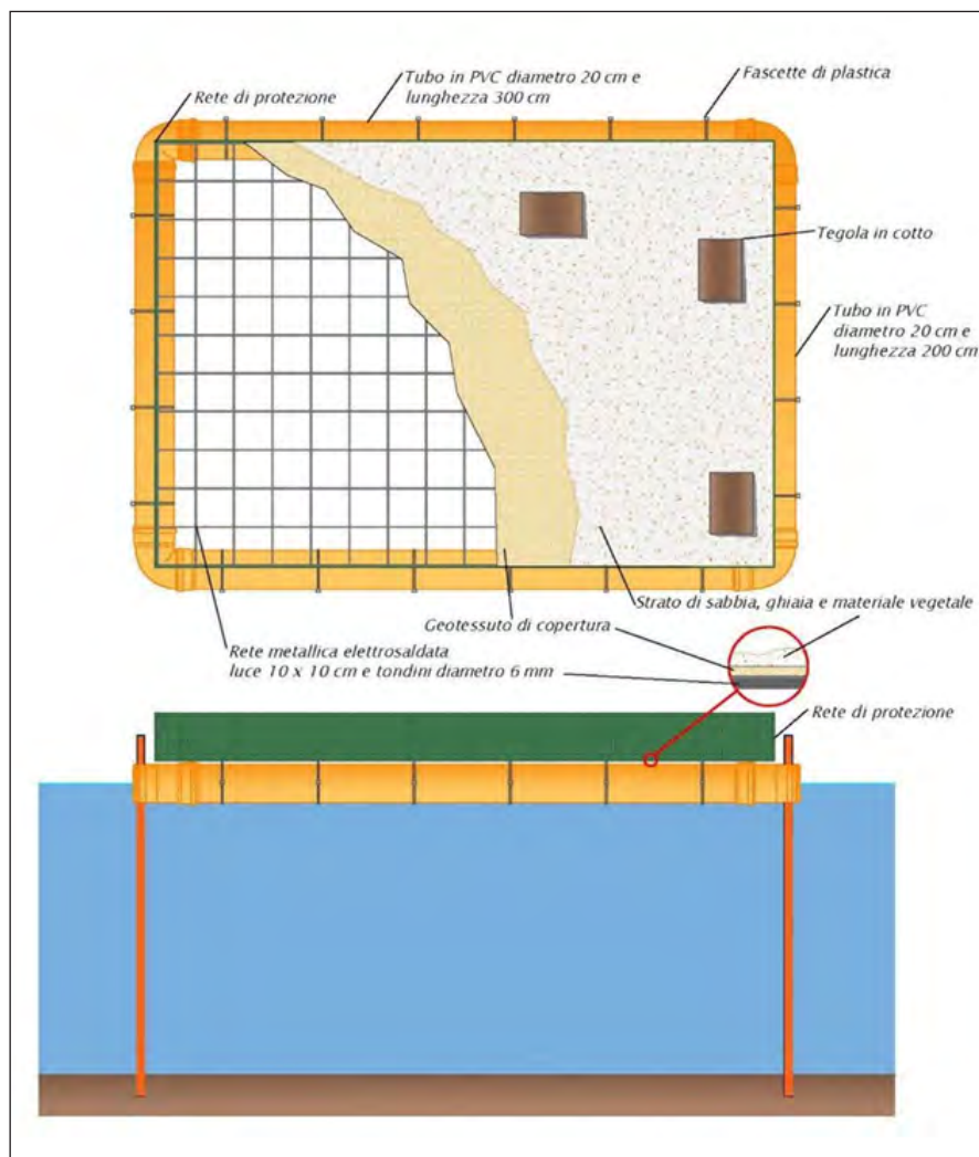
Schema realizzativo di una zattera per la nidificazione di limicoli e sterne
